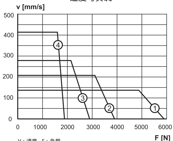
速度与负载
