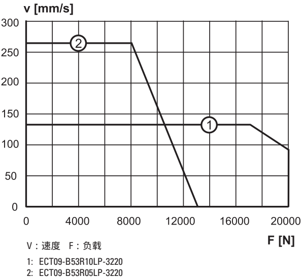
速度与负载
