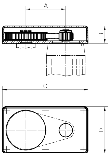
BGM09/41/81 - 无U形夹选件
