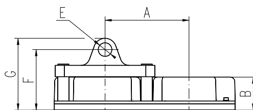
BGM81 - R型U形夹选件
