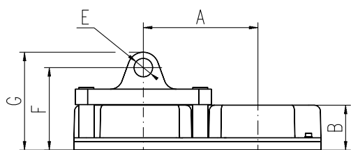
BGM09/41/81 - S型U形夹选件
