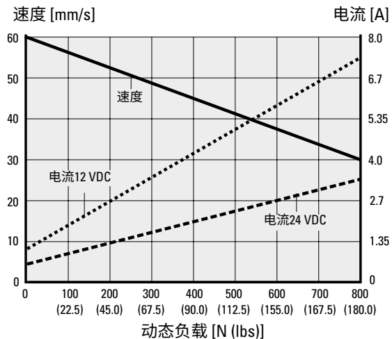
滚珠丝杠型 (MX • • B)
