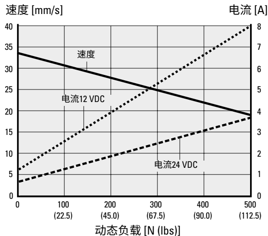
梯形丝杠型 (MX • • W)
